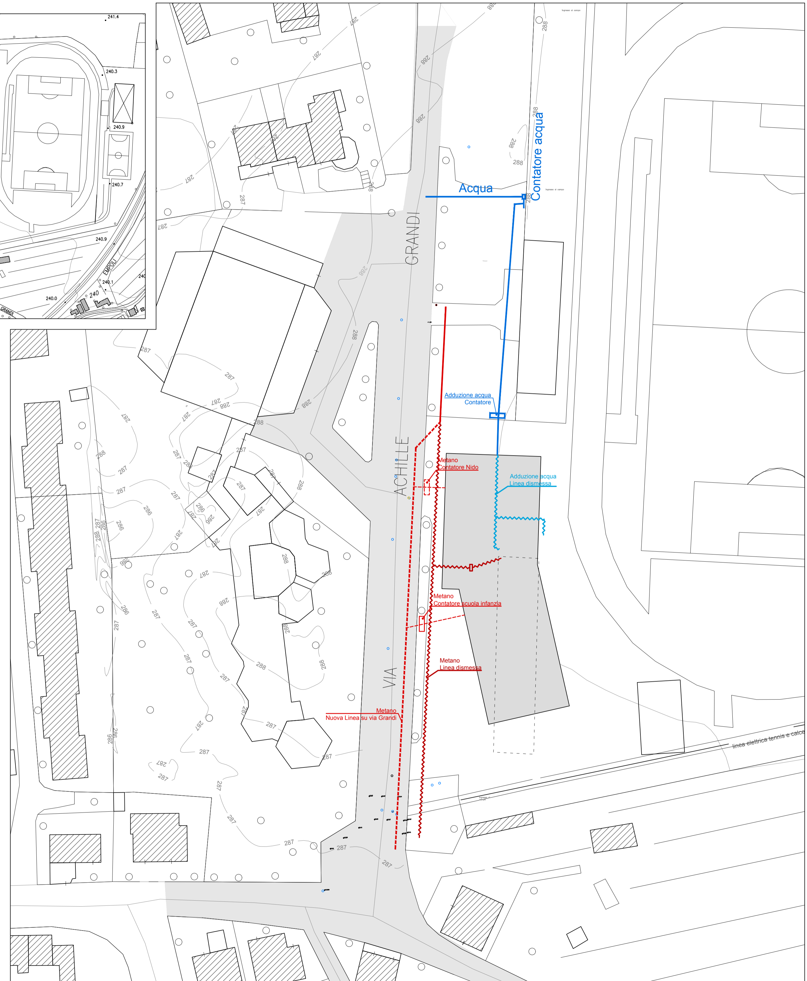
Planimetria stato modificato - scala 1:500
