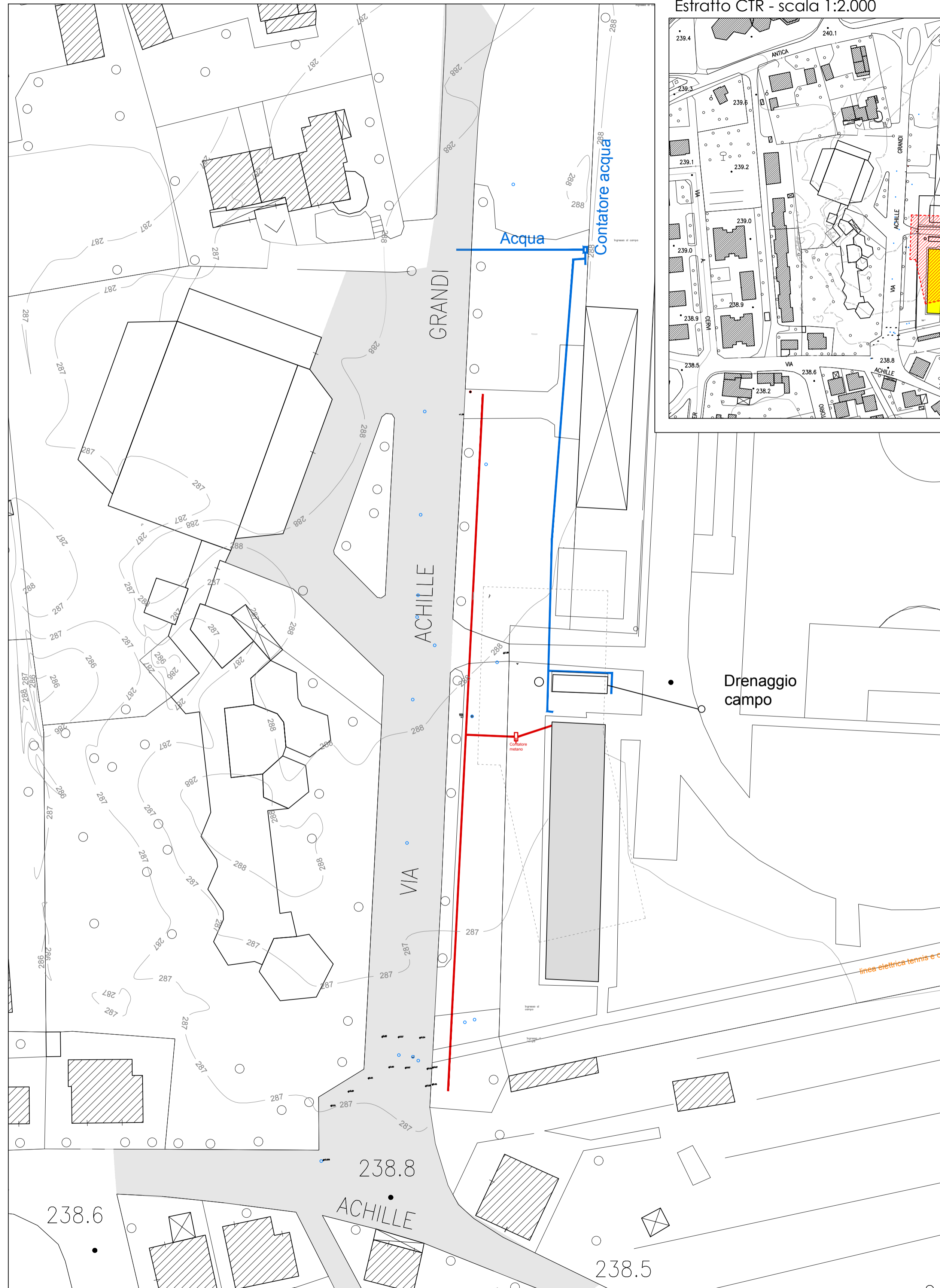
Planimetria stato attuale - scala 1:500
